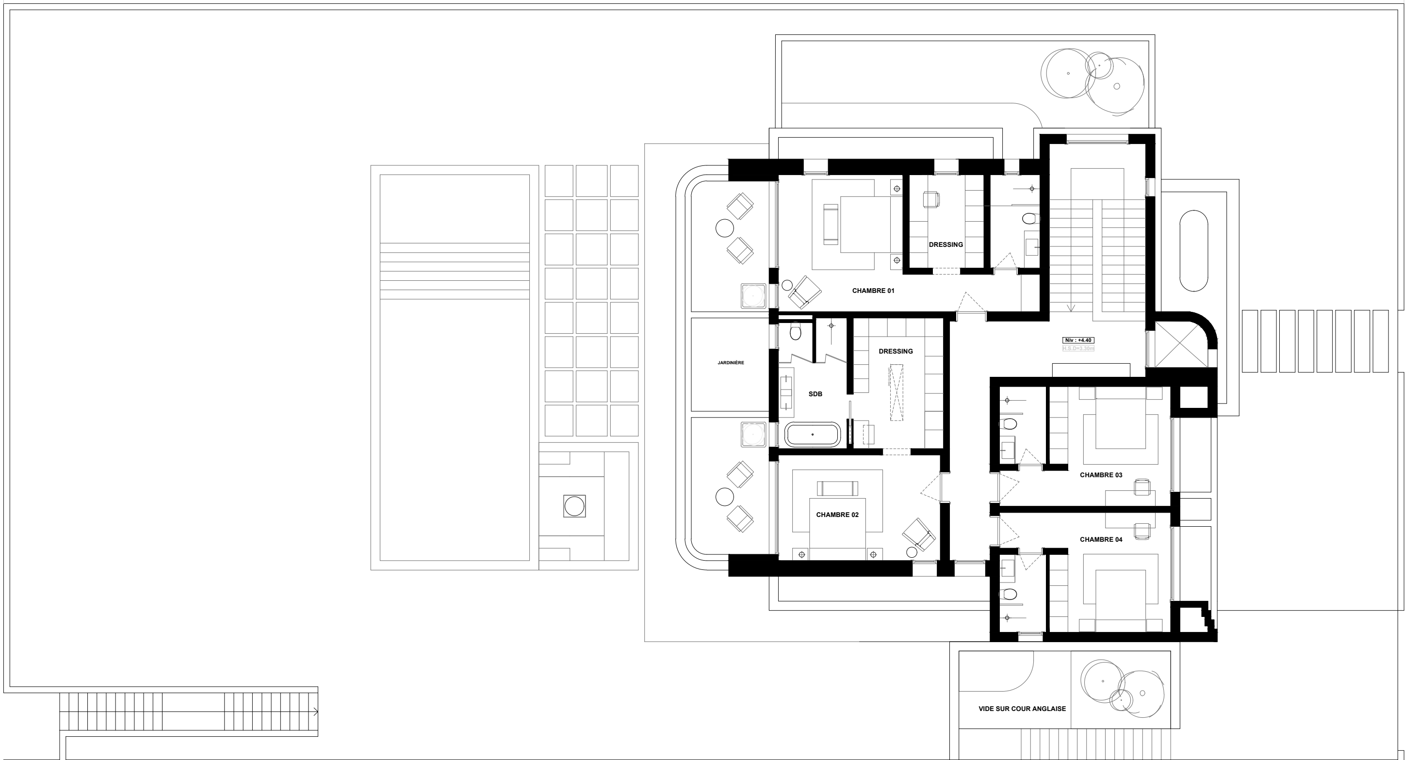
02 — PLAN ETAGE
