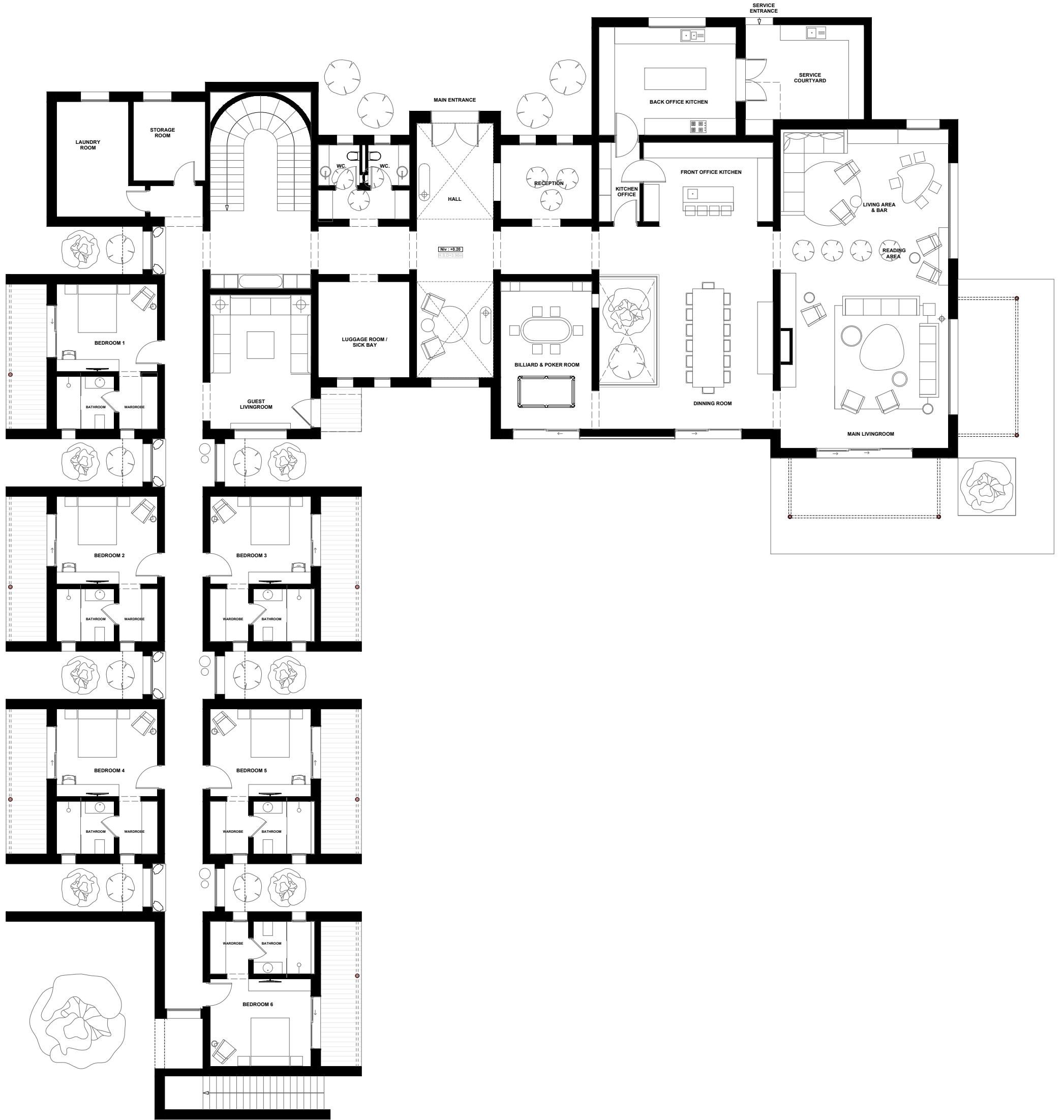
01 — PLAN RDC
